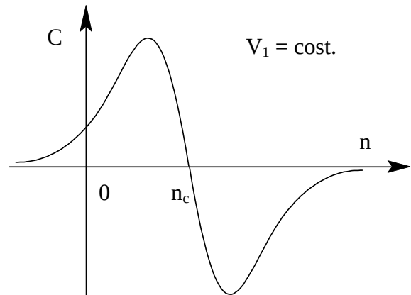
Caratteristica meccanica di una macchina asincrona in funzione del numero di giri
