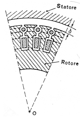
Doppia gabbia per rotore di macchina asincrona.
